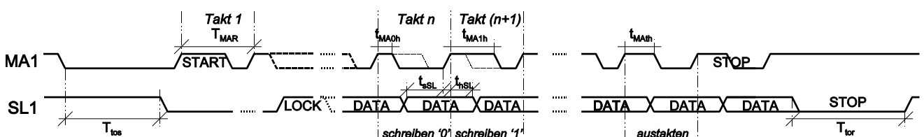
Bild 9: Zeitdiagramm Registermodus
