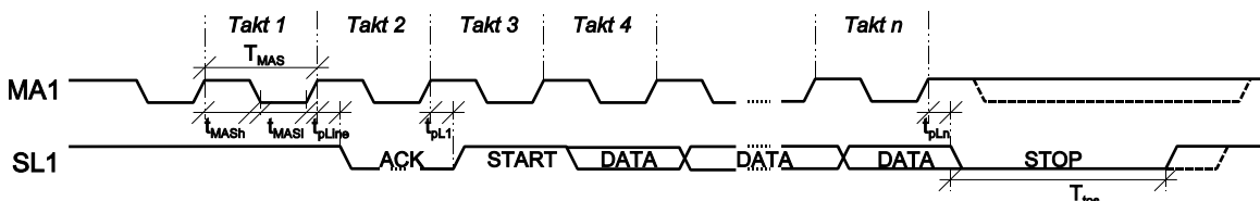
Bild 8: Zeitdiagramm Sensormodus
