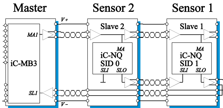
Bild 13: Beispielkonfiguration
