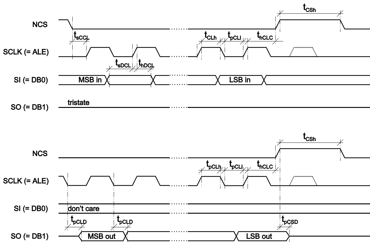
Bild 7: \mu C-Schnittstelle im SPI-Modus, Schreibzyklus (oben), Lesezyklus (unten)
