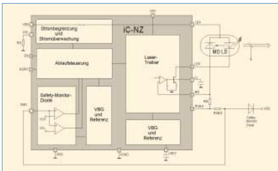
Bild 1: Einfehlersichere Laserdiodenansteuerung mit dem iC-NZ
